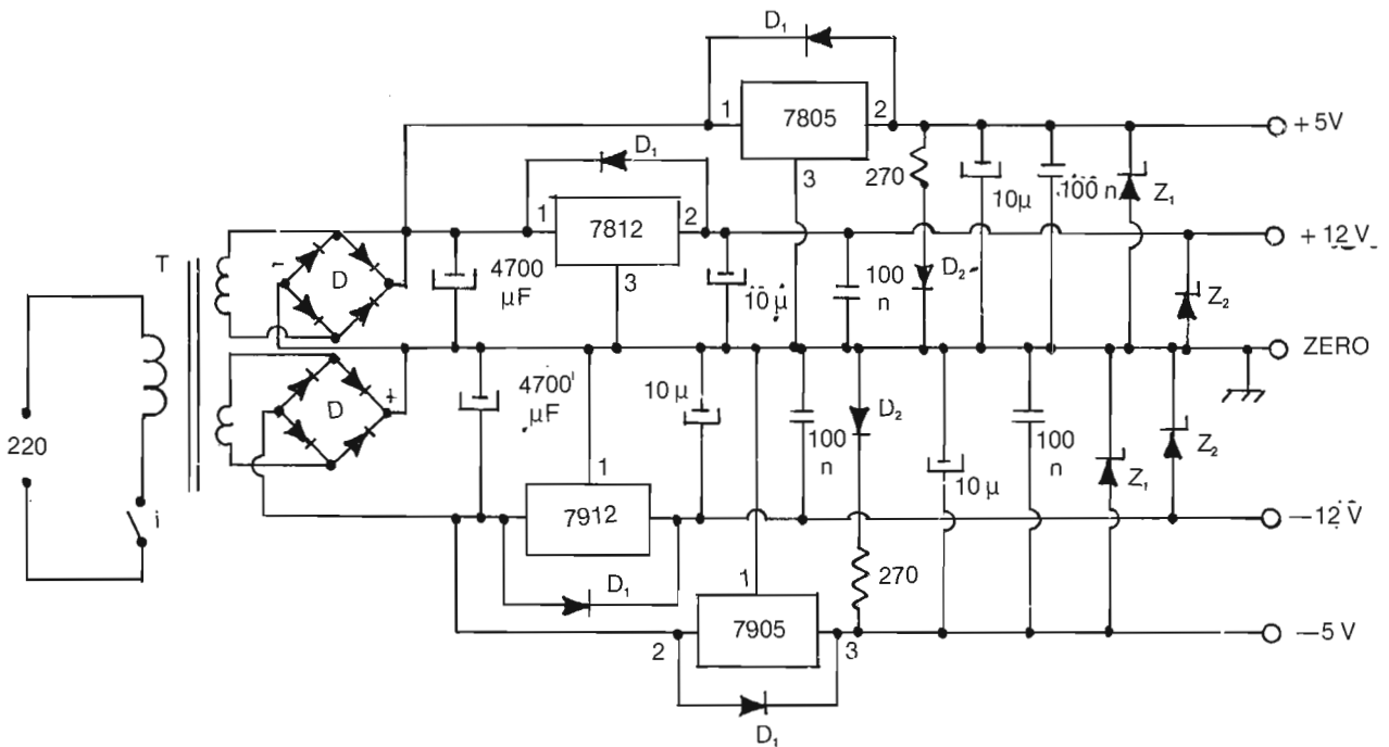
Fig. 4 - Un alimentatore da 2 A con tensioni \pm 12V e \pm 5V . D = Due ponti di diodi da 12V/2A di lavoro ad es. mod. B40-C1500 D1 = Quattro diodi al silicio 1N4001. D2 = Due LED - uno rosso l'altro verde Z1 = due Zener da 6,8 V Z2 = due Zener da 15 V T = Trasformatore da 35 W lordi Regolatori di tensione: 7812 positivo 12 V; 7805 positivo 5 V 7912 negativo 12 V; 7905 negativo 5 V nota: i condensatori da 100 nF sono ceramici; quelli da 10 \mu F al tantalio, gli altri: elettrolitici.
