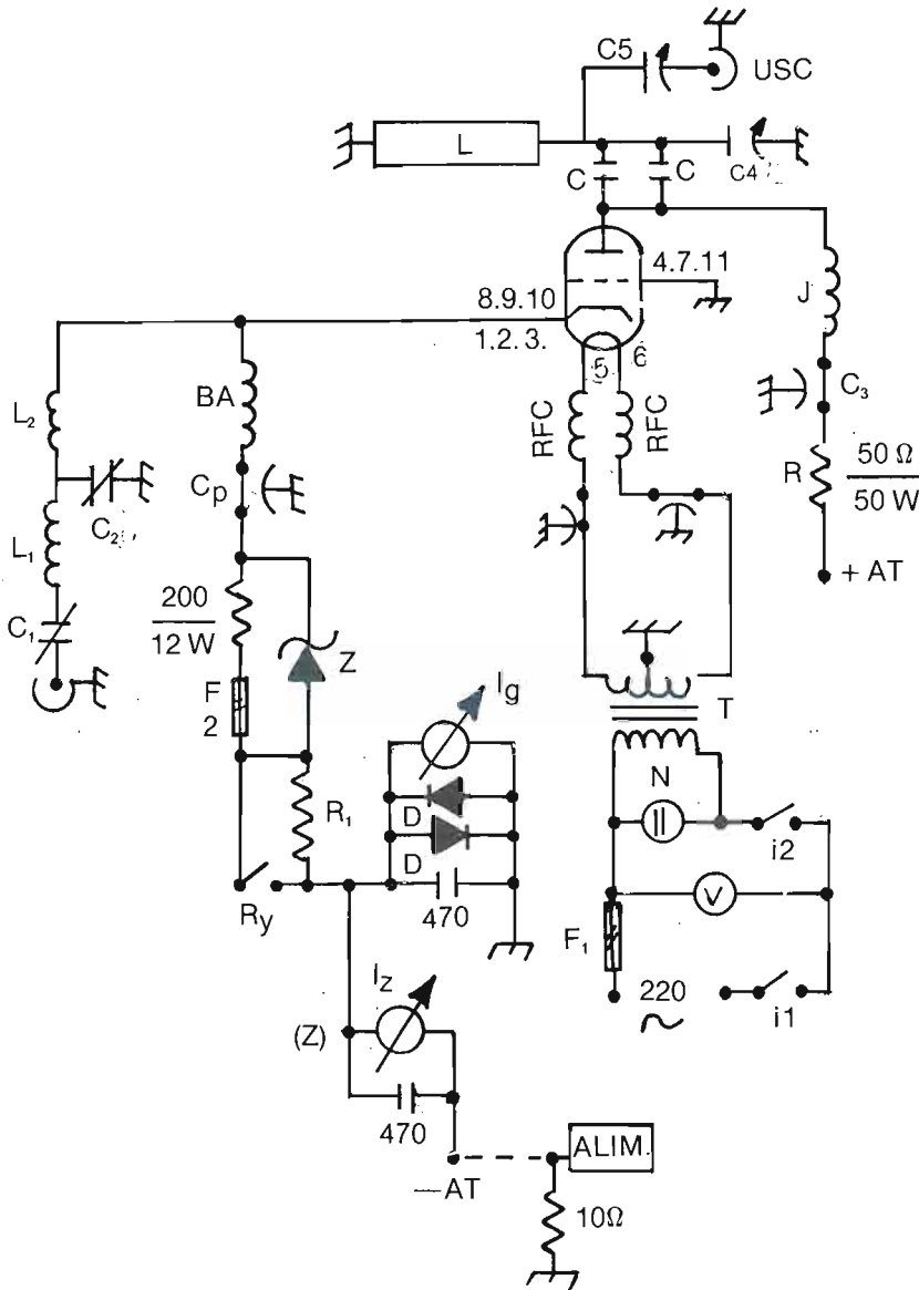
Fig. 2 - Schema elettrico del P.A. con triodo «3C x 800A7». C1 = C2 = Variabile ad aria 14 pF = Johnson 189-505-4; o simili C3 = passante per alta tensione — ERIE 1280/060 = 1,5nF/2,5 kV C4 = C5 = piattelli Ø 35 mm d'ottone-Vds. testo Cp = condensatori passanti 1nF/500V = ERIE 357-001 C = due ceramici barilotto da 500pF/7,5 KV L1 = 8 sp. filo 1,5 stagnato Ø int 10 lungh. avv. 18 mm L2 = 5 sp. filo 1,5 stagnati Øi 10 lungh. avv. 13 L = linea in piatto d'ottone 3,5 x 21 cm; spess. 1,5 mm BA = 35 sp. filo 0,5 sm. non spaz. Ø int = 4,5 lungh. 18 mm RFC = due bobine di 11 sp-filo 1 mm/smalt; Ø interno 1 cm J = 10 sp. filo 1,5 stagnato Ø int 13 mm; lungh. avv. 3 cm R1 = 10 KΩ—12W: riduce I g in stand-by Z = diodo Zener 5,1 V — 10 W = 1N3996A D = diodi 1N4001 F1 = fusibile da 2A F2 = fusibile da 1,5A N = lampada segnalaz. al neon con resistenza per 220 V V = Ventola da 25 CFM con motore 220V T = Trasfo da 35W-lordi. Sec da 13,5V-2A con presa centrale I g = 100 mA fondo scala; I a = 5 volt f.s.; 2 strumenti da 1 mA Ry = contatti relay norm. aperti (ricezione). La bobina del relay si eccita a comando VOX o con la s.f. del pilota.
