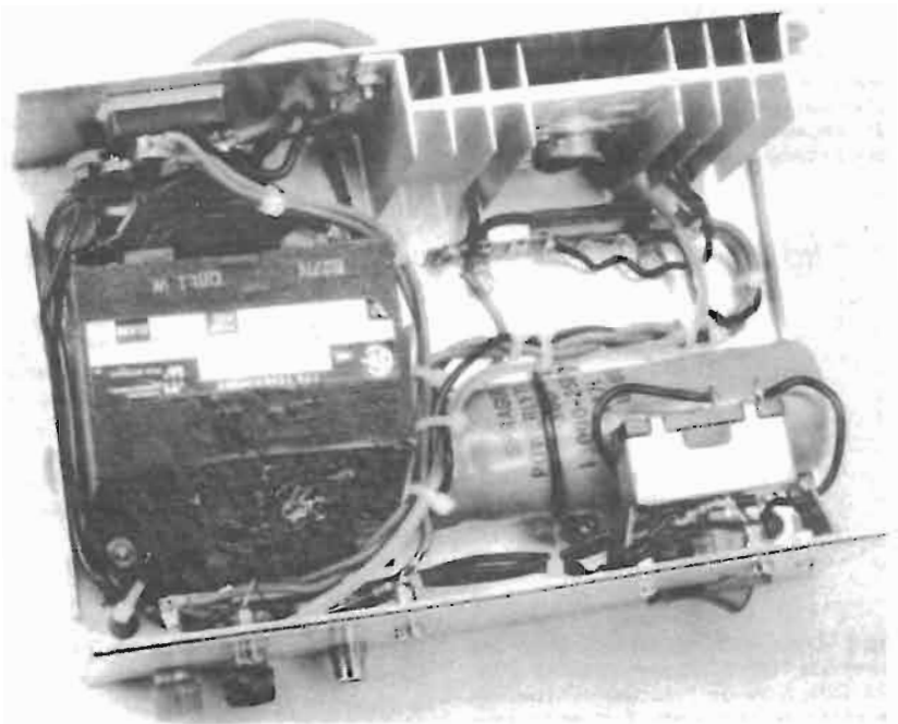
Fig. 3 - La realizzazione dell'alimentatore da 5 A. Si osservi il grosso dissipatore di calore a cui è fissato il regolatore di tensione. Nonostante questo, se si richiede una tensione minore di 13 V; può darsi che la potenza dissipabile diventi eccessiva — in tal caso una protezione interna al regolatore interrompe l'erogazione.
