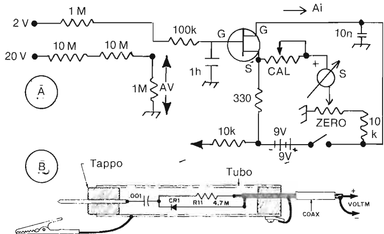
Fig. 1 - A) Voltmetro elettronico con un FET. Sono previsti due ingressi c.c. a 2 e 20 V ma se si usa solo una R da 10 M \Omega si ha un fondo scala di 10 V e con 40 M \Omega il f.s. diventa 40V. L'alta impedenza d'entrata rende lo strumento molto utile. Il JFET è un modello qualsiasi d'uso generale in a.f. I potenziometri CAL e ZERO sono da 2500 \Omega ; ZERO è un TRIMMER.
