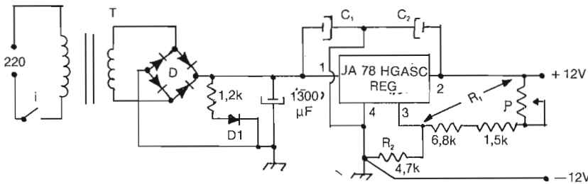
Fig. 1 - Schema elettrico dell'alimentatore da 5 a 20 volt, con erogazione di corrente 5 amperre.
