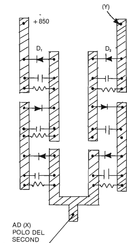
Fig. 9 - Costituzione delle due serie DRC per il circuito duplicatore di tensione. Rif. figura 7C. Le combinazioni su circuito di vetronite formano F1 e D2 della citata figura; ad essa si riferiscono anche le indicazioni dei terminali (X) (Y).
