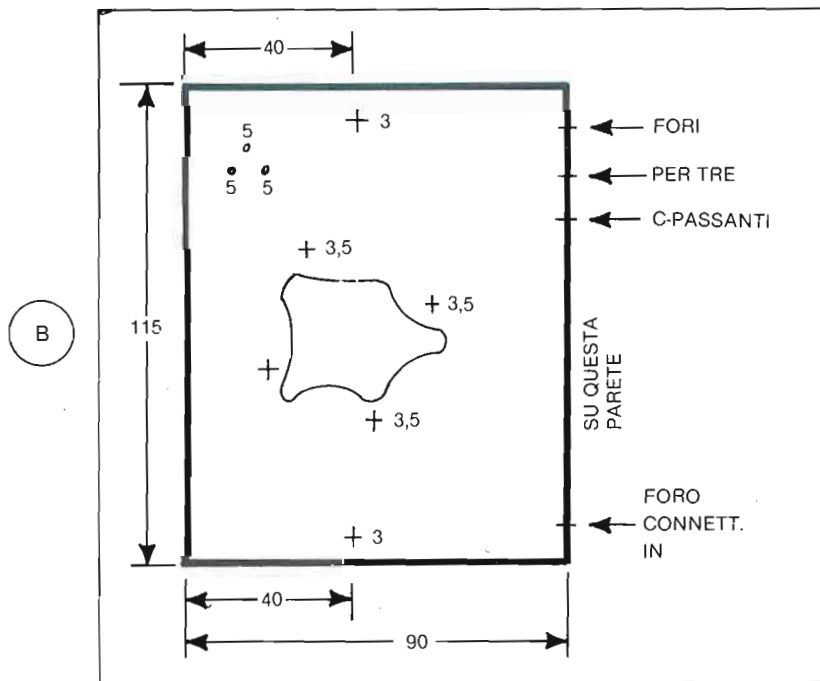
Fig. 7 - La box di catodo è alta 25 mm — i riferimenti sono rappresentati dai tre fori di 5 mm disposti a triangolo — per la sua aereazione. Il fondo della box è applicato al fondo della cassetta anodica, la finestra per lo zoccolo praticato su questo fondo deve coincidere con l'altro. Le due cassette sono unite con le viti i cui fori sono indicati. I due da 3 mm in alto ed in basso sono per le viti che oltre a migliorare l'unione, sostengono le colonnette laterali (di teflon) alle quali si assicura la periferia del collare anodico. Nel coperchio della box vi sono due fori per la regolazione di C1 e C2 — da questi fori esce anche l'aria di raffreddamento (Vds fig. 5B).
