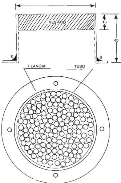
Fig. 8 — Il camino, applicato ad un foro di 70 praticato nel coperchio della scatola anodica in corrispondenza del triodo. Alla estremità opposta del coperchio, vi è il foro per la ventola. Dal camino uscirebbe non solo aria calda ma anche un bel po' di alta frequenza. Il filtro per l'arresto dello spillamento a.f. è costituito da una specie di «vespaio» formato da 145 tubicini di rame 4 x 3 affiancati. Ciascun tubicino è lungo 13 mm. I tubicini sono pressati entro il foro interno del camino e fermati con un collante per metalli che resiste al calore (UHU a due componenti). L'effetto di attenuazione in dB è dato dalla relazione:
