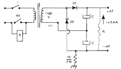
Fig. 10 - Un alimentatore duplicatore economico
