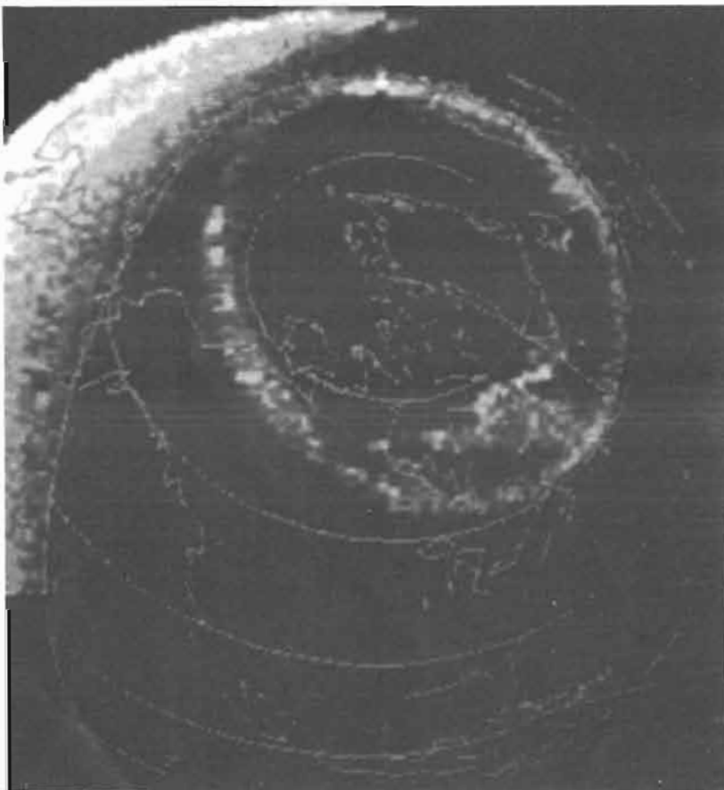
Fig. 2 - Dal 1981 il Dynamics Explorer 1° in orbita ellittica-polare ci consente di visualizzare le Aurore. Non più immagini da fantasia, ma immagini reali.
