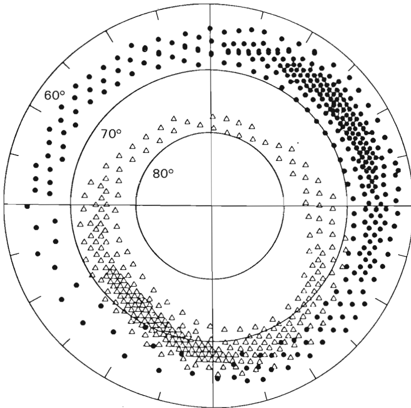
Fig. 3 - L'aurora visibile s'innesca dove più intensa è la precipitazione di particelle. Quindi l'ovale aurorale con sole in attività normale, sta fra il 75° N g ed il 65° N g . Le rilevazioni riometriche indicano che le precipitazioni nell'ovale sono di due tipi: «a pioggerella» (punti) ed «a spruzzi» (triangoli). I due tipi di precipitazione come si vede nella figura (dalla relazione di Hartz & Brice) hanno distinte collocazioni latitudinali e temporali. Di giorno prevale «lo spruzzo»; di notte «la pioggerella» ma vi sono ore in cui i due tipi si sovrappongono.
