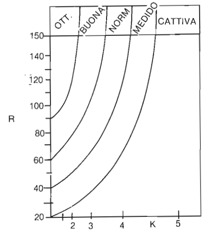
Fig. 7 - Grafico di correlazione fra indice k e propagazione. Anche se un R elevato fa prevedere una eccellente propagazione; per numerosi giorni al mese, a causa dei flares e dell'alta temperatura coronale, si può avere un «vento» al di sopra dei livelli medi che provoca perturbazioni magnetiche. Un indice k maggiore di 2-3 è già in grado di deteriorare la propagazione HF, anche nei momenti migliori. Oggi con propagazione «mediocre» in ogni caso, una leggera perturbazione magnetica è già in grado di far scendere le condizioni a «cattive».
