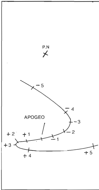
Fig. 8 - A causa della rotazione degli apsi, la curva per il tracciatore di OSCAR 10 ha assunto ora, questa forma.
