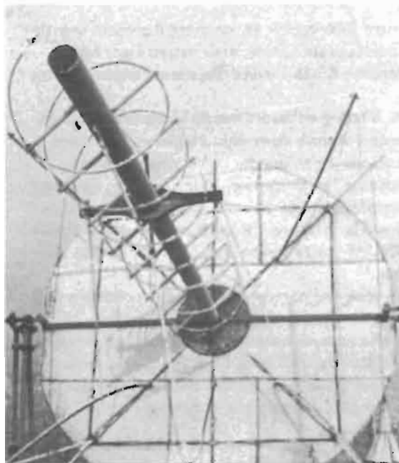
Fig. 5 - La soluzione per il «modo A» del telescopio DJ7AA. Una spirale per i «due metri» davanti ad un disco riflettore del diametro di 2,60 m. A distanza critica dal riflettore è tesato il quadrato di filo lungo una \lambda che costituisce la «quad» per i 29 MHz.
