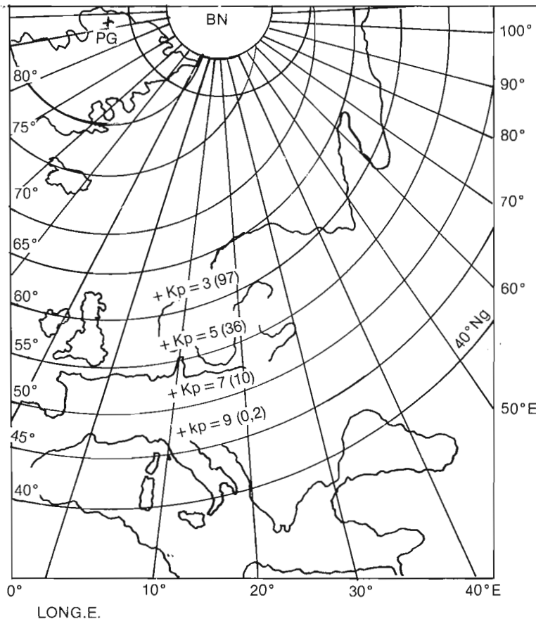
Fig. 5 - Quando l'attività solare ed in particolare il «vento» è al di sopra dei valori medi, il campo geomagnetico è perturbato, ed i suoi indici sono maggiori di k = 2 .
