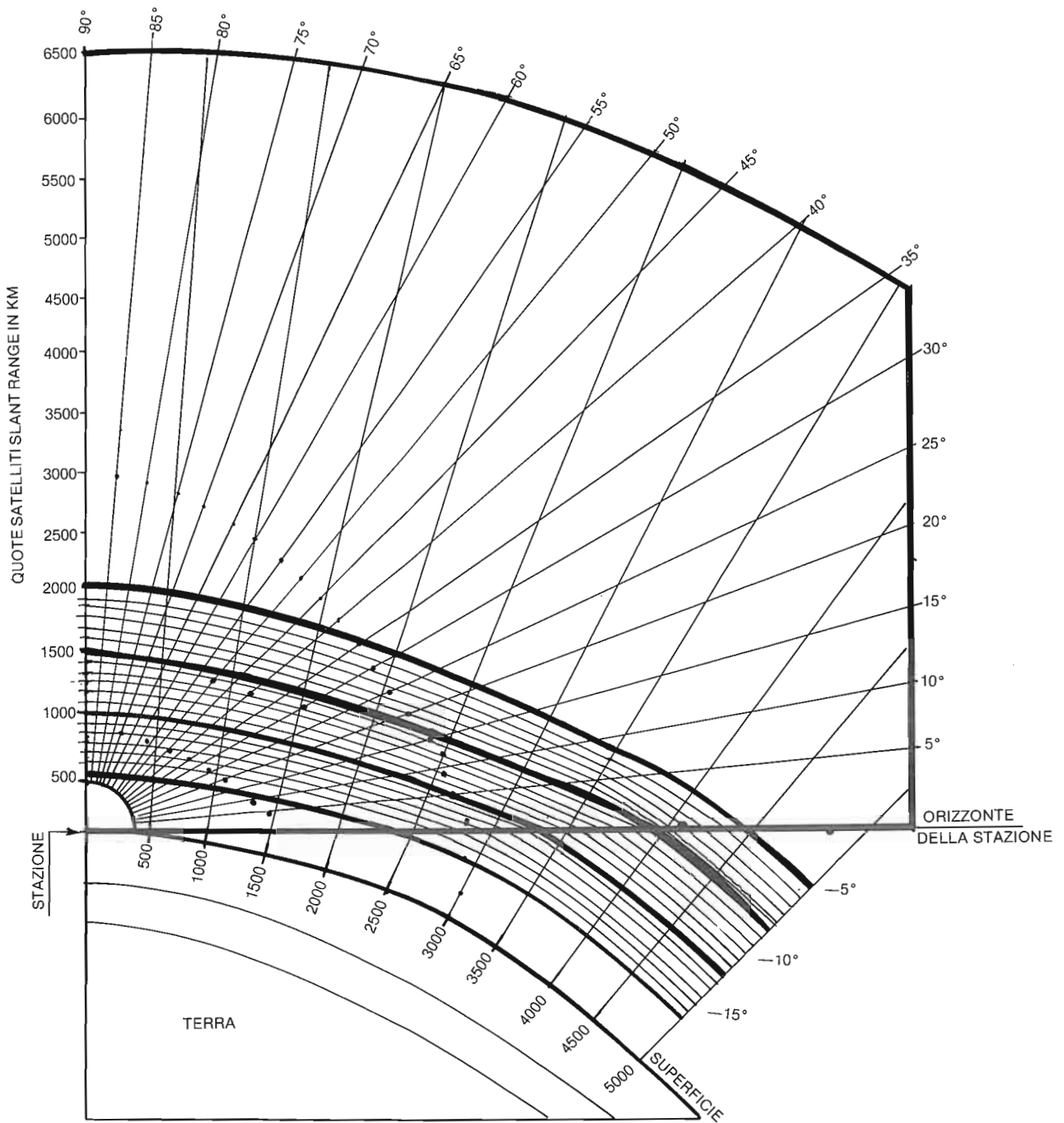
Fig. 2 - Il raggio del cerchio d'acquisizione dipende dalla quota del satellite. I punti AOS e LOS si trovano alla max circonferenza del cerchio ideale che circonda il proprio QTH. Per il max AOS = momento in cui il satellite compare all'orizzonte visto dalla propria antenna, occorre che la sensibilità del sistema ricevente sia la max praticamente possibile. Se un satellite in orbita circolare ha la quota di 1700 km il raggio del cerchio è 4300 km quindi in un'orbita molto vicina al proprio QTH avremo una distanza fra AOS e LOS = al diametro del cerchio ossia maggiore di 8000 km. LOS = perdita del segnale: quando il satellite tramonta all'orizzonte.
